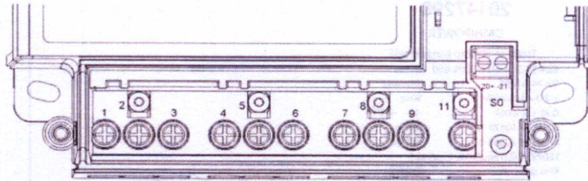
Slika 5. Nacrt priključnice brojila
