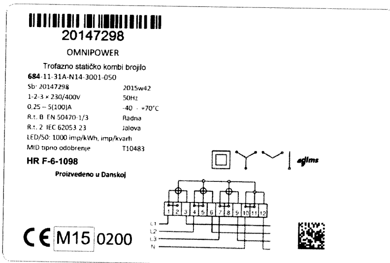
Slika 7. Natpisna pločica
