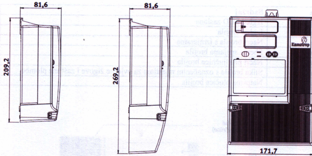
Slika 3. Nacrt brojila s izmjerama
