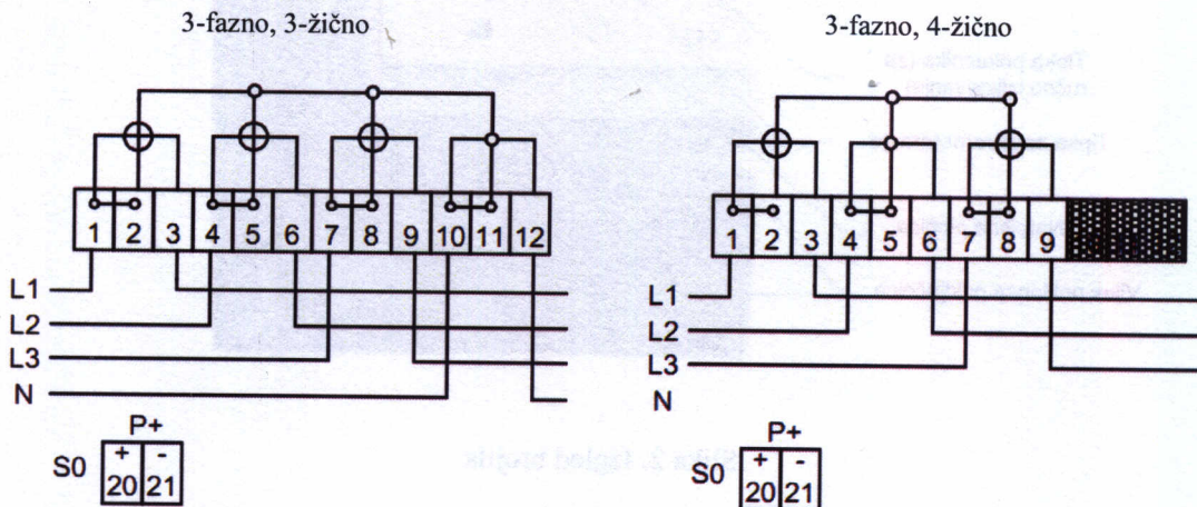
Slika 4. Shema spajanja
