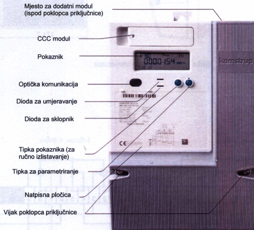
Slika 2. Izgled brojila
